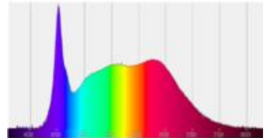
Spektrale Strahlungsverteilung im Bereich 180 - 800 nm
